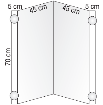
Rückansicht mit Saugnäpfen als Befestigung
